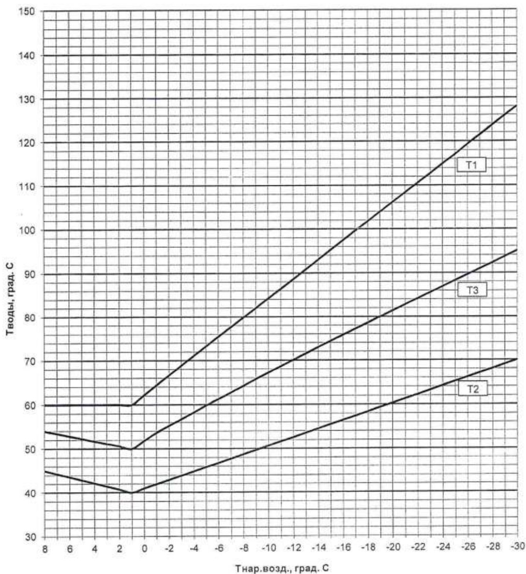
Температурный график отпуска тепловой энергии от Апатитской ТЭЦ на г. Апатиты на 2024-2025 гг.
