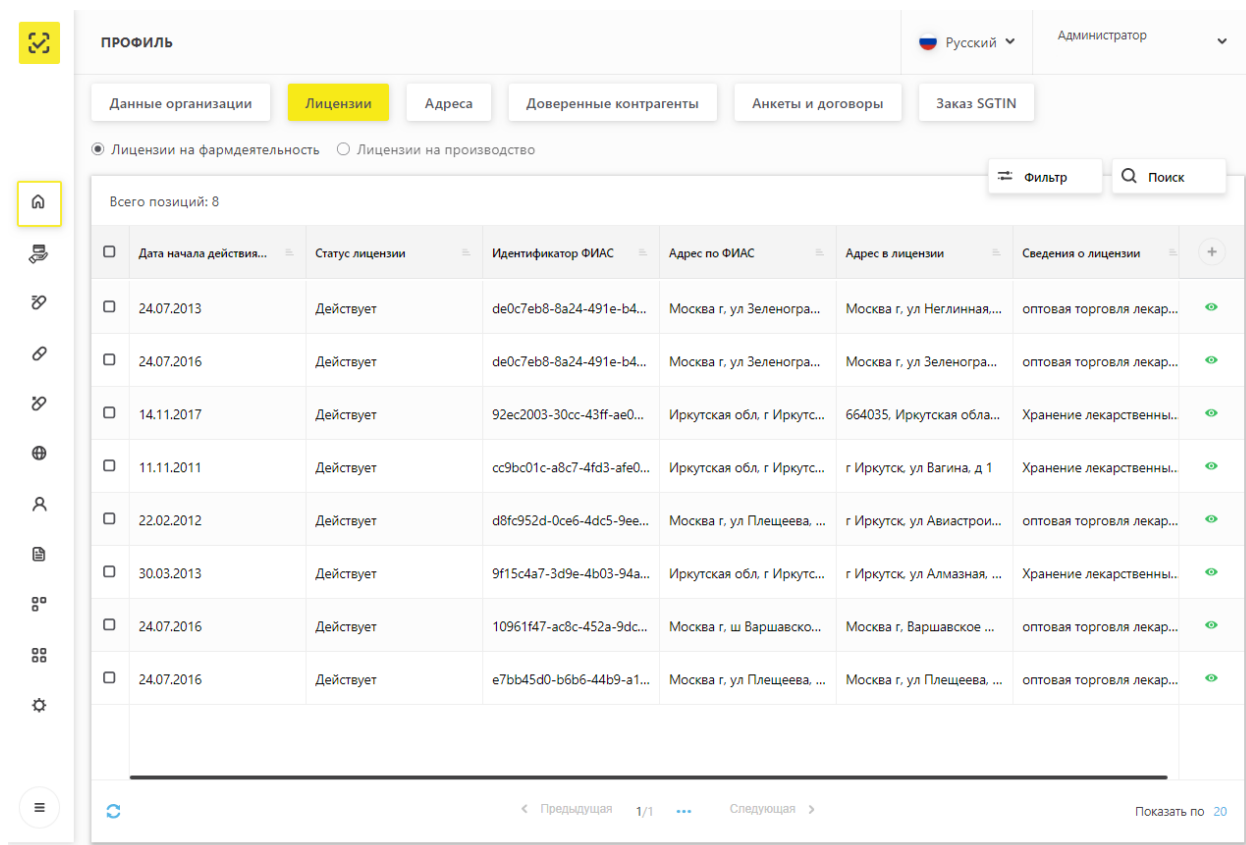
Рисунок 23 – Вкладка Лицензии
