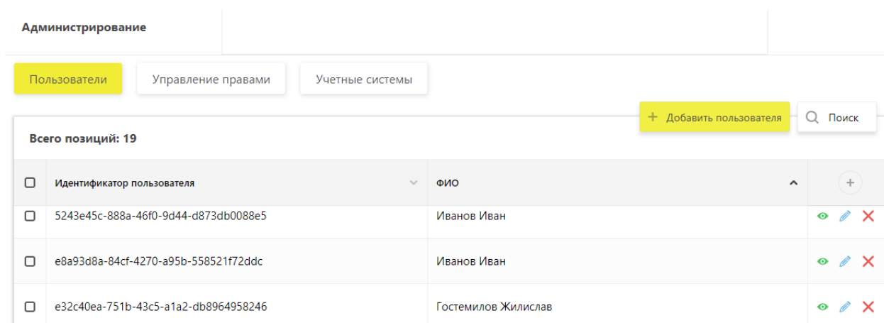
Рисунок 111 – Вкладка Пользователи
