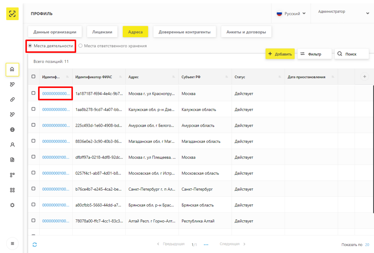
Рисунок 173 – Выбор МД
